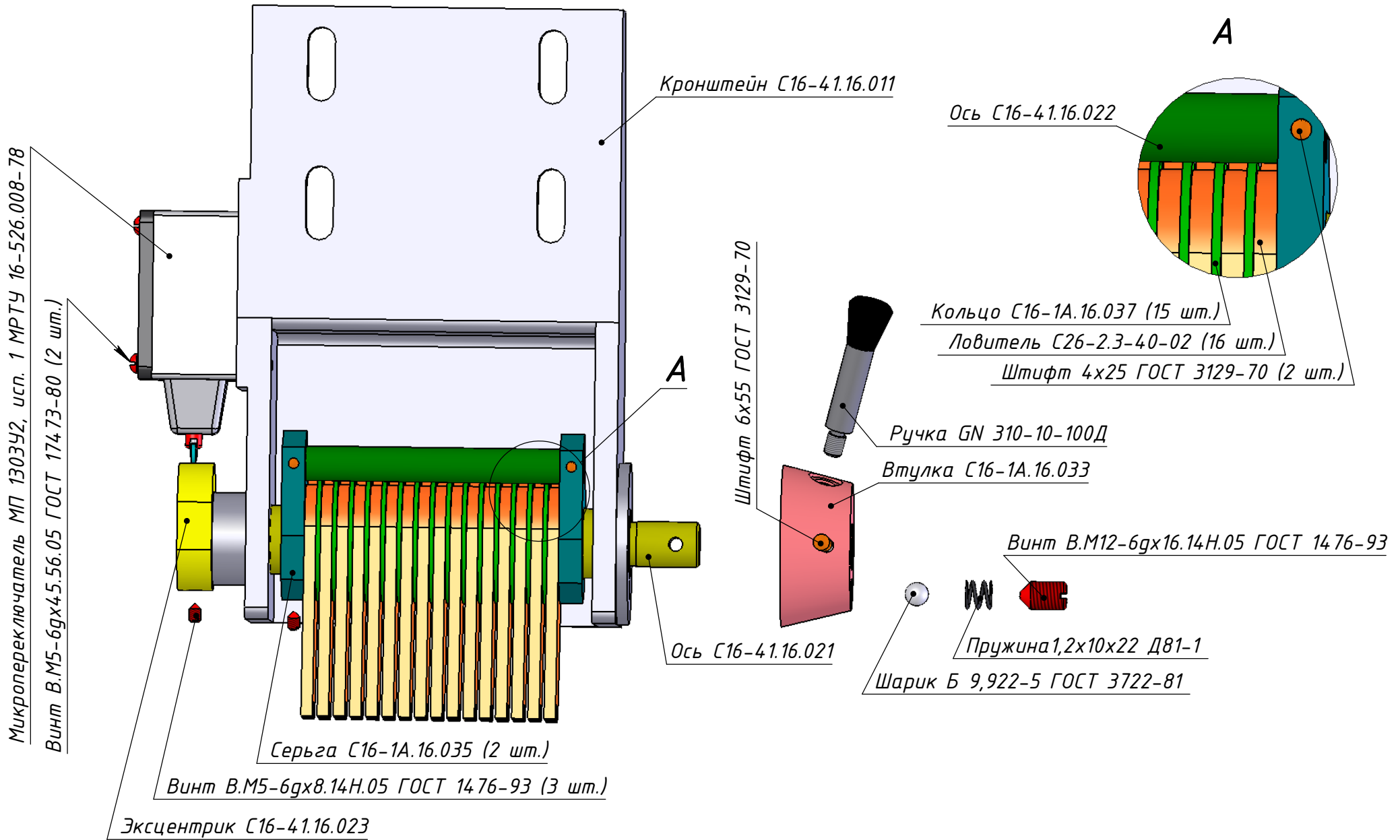
Козтевая защита С16-4.1.16.000 СБ (Лист 3/3)
