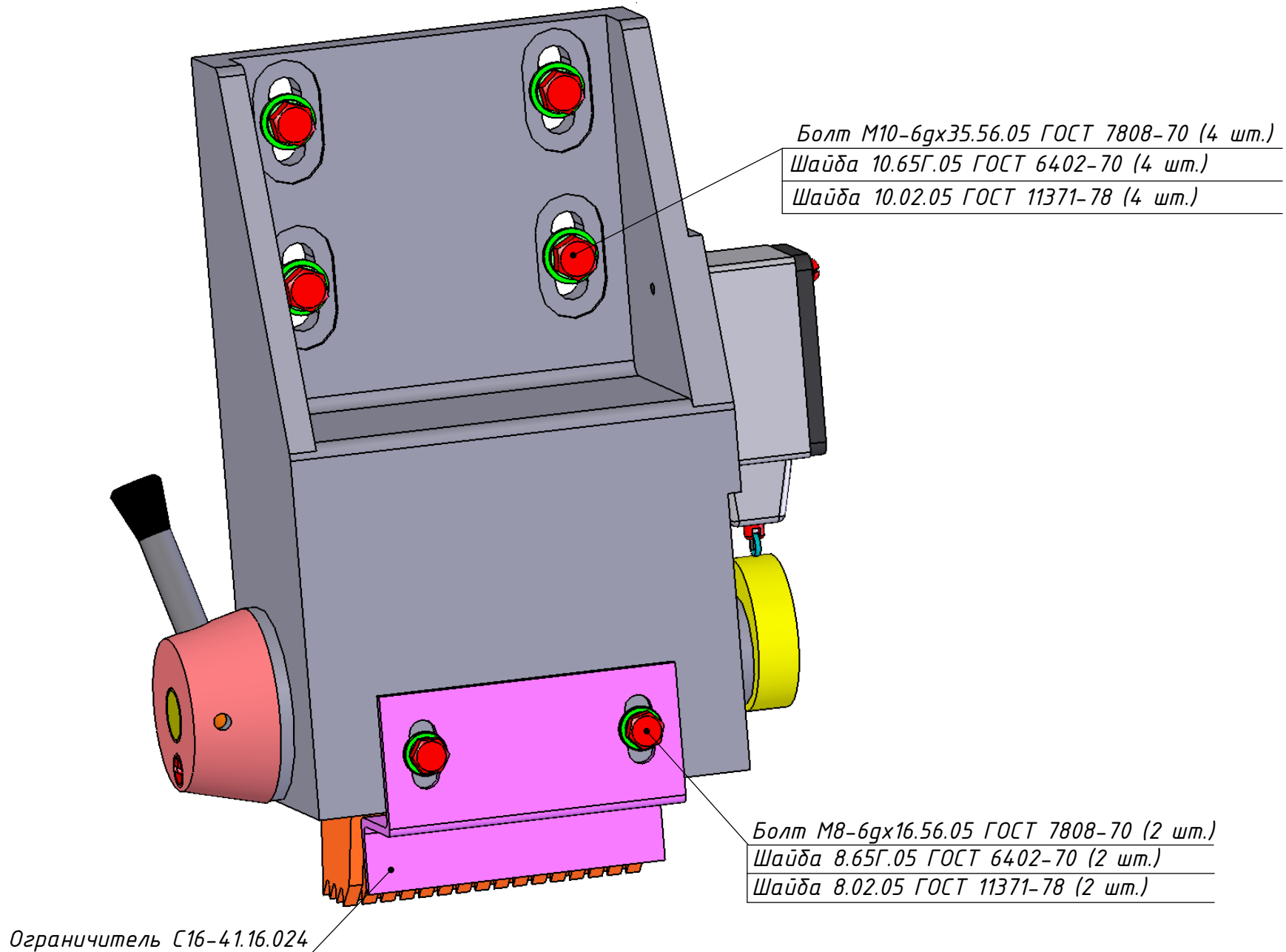
Козлевая защита С16-41.16.000 СБ (Лист 2/3)
