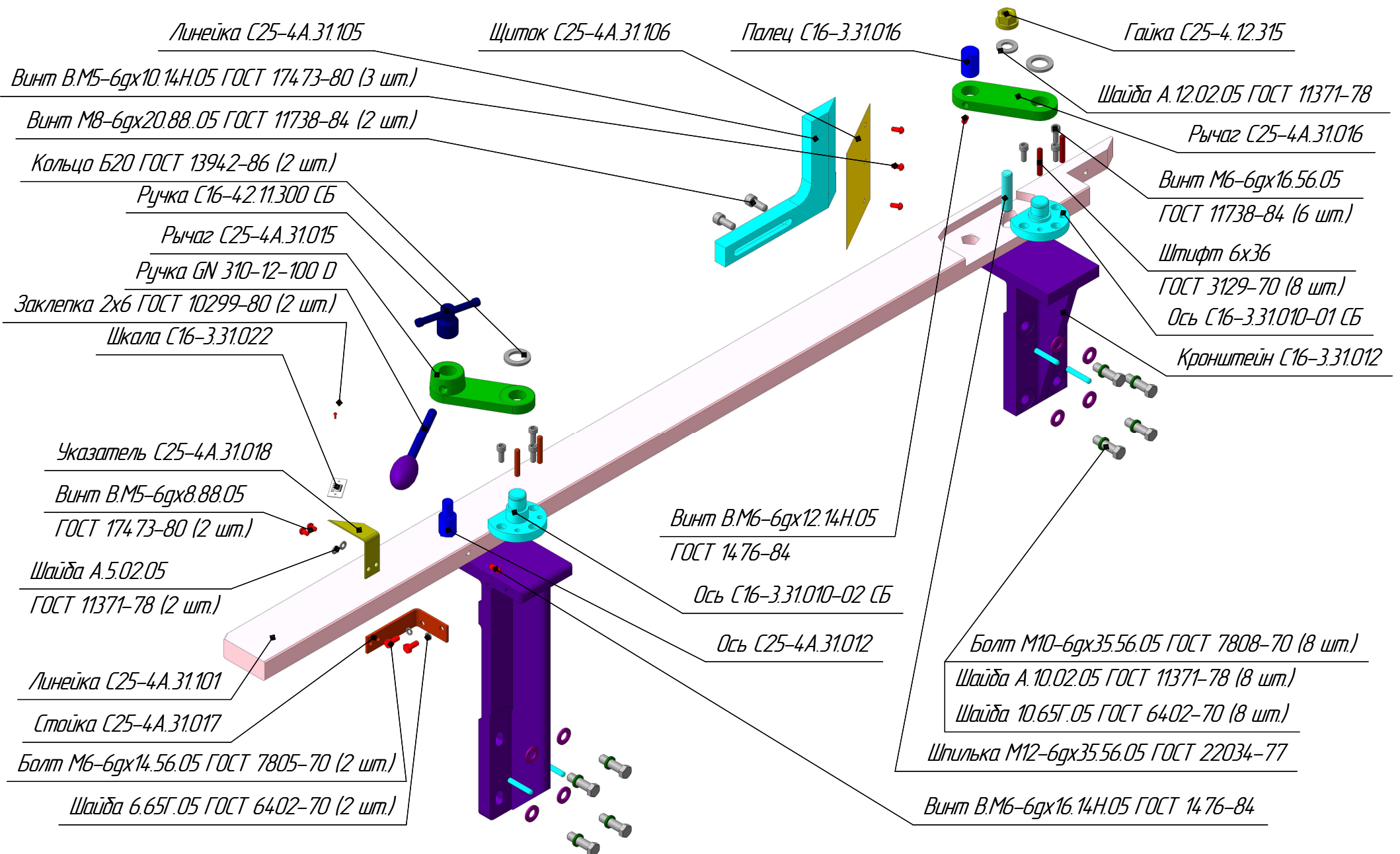
Линейка С25-4А.31.000 СБ (Лист 2/2)
