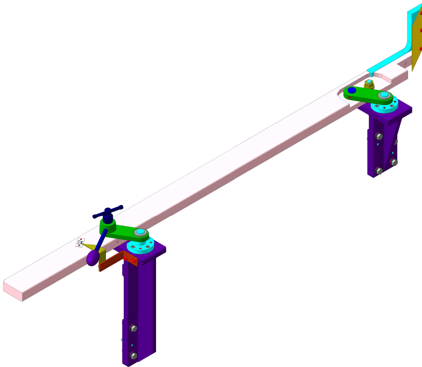
Линейка С25-4А.31.000 СБ (Лист 1/2)
