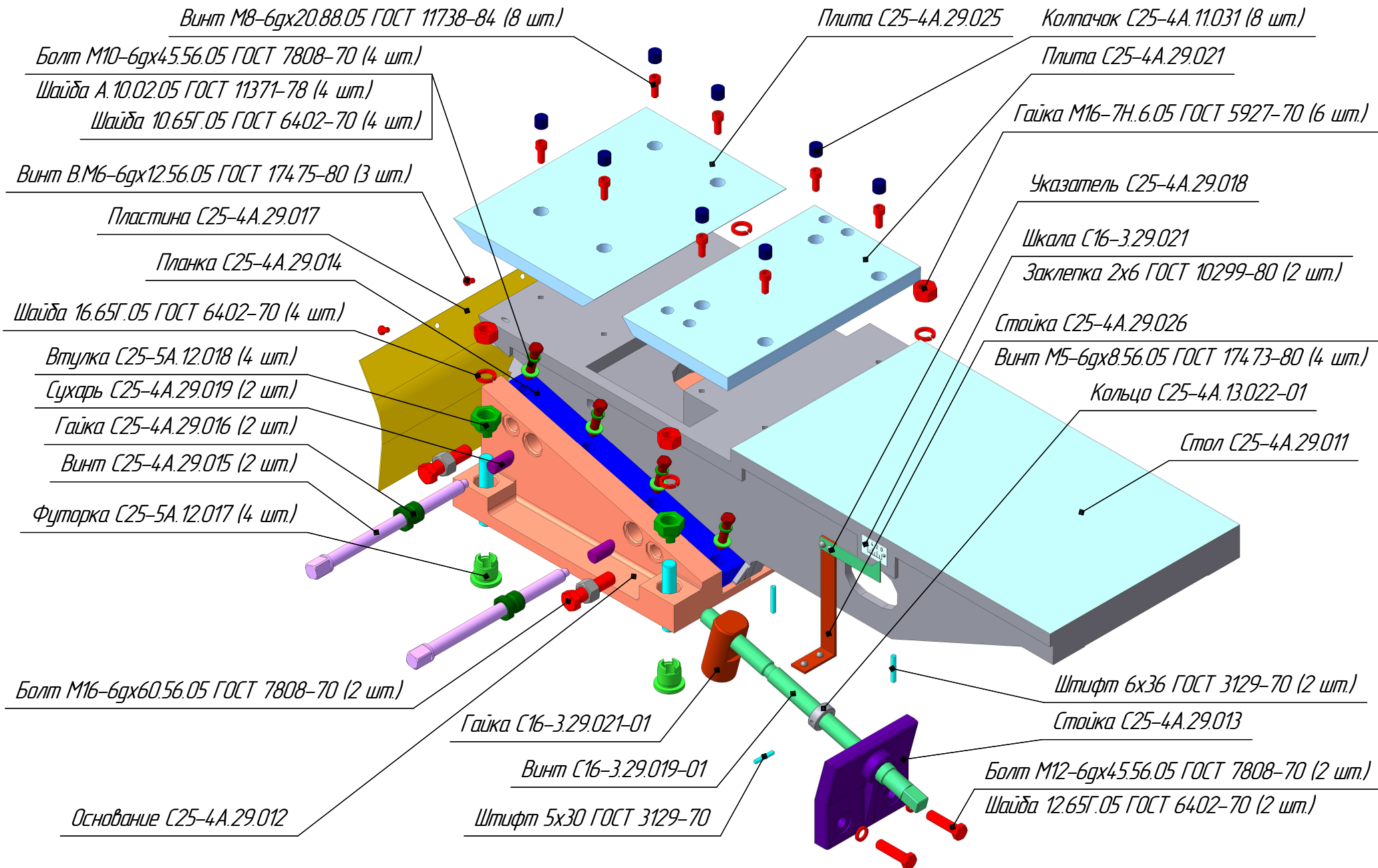
Стол передний С25-4А.29.000 СБ (Лист 2/2)
