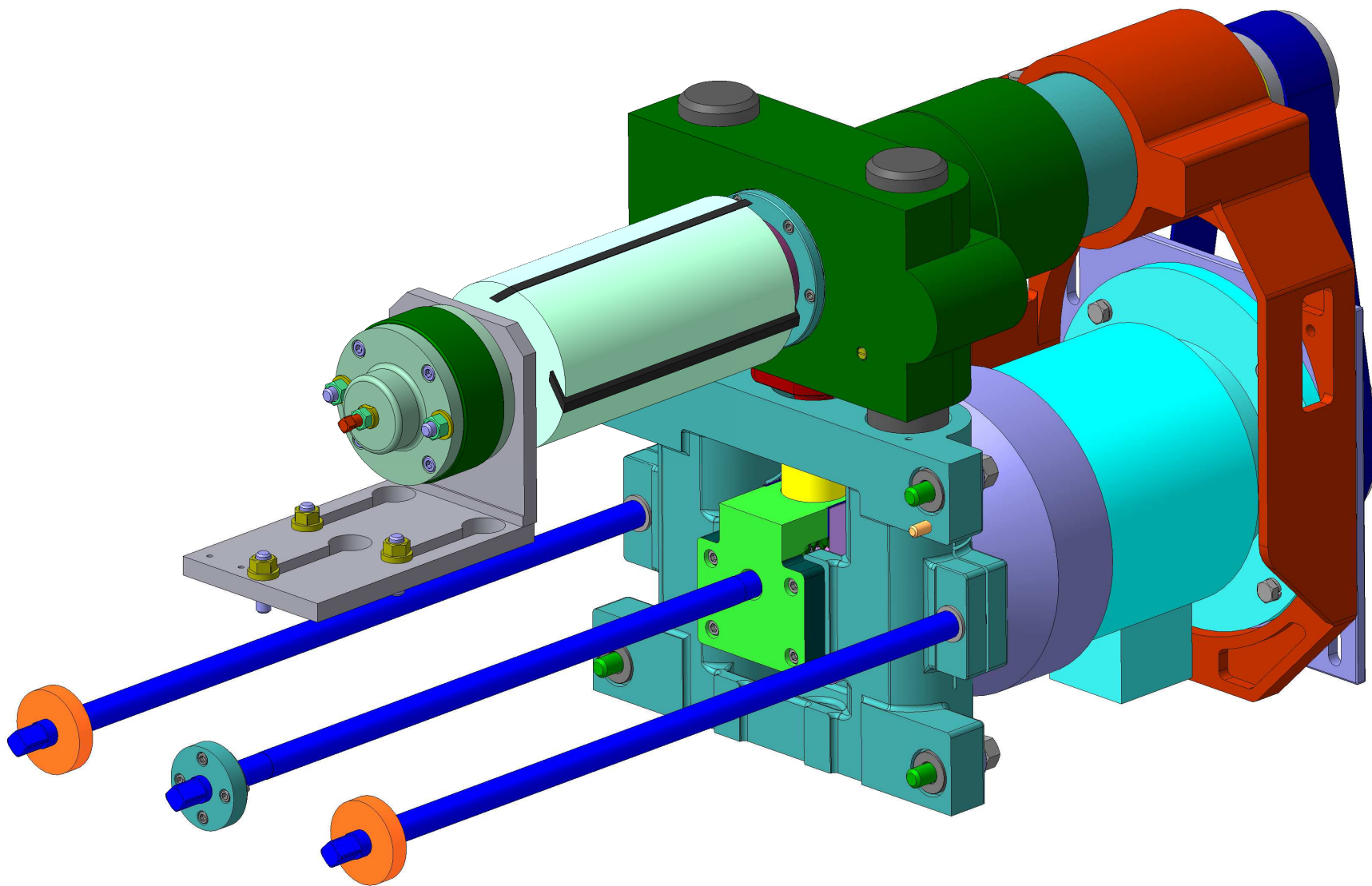
Суппорт нижний С25-4А.12.1.000 СБ (лист 1/7)
