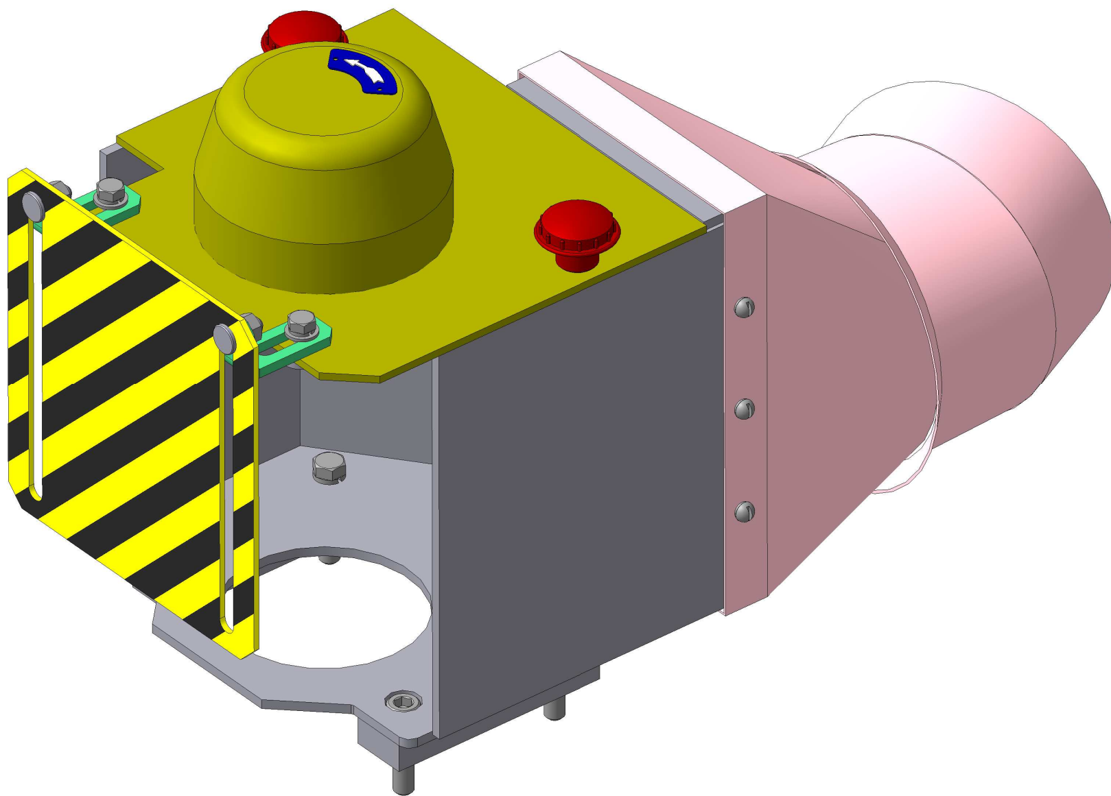
Ограждение С25-4А.13.100 СБ (лист 3/6)
