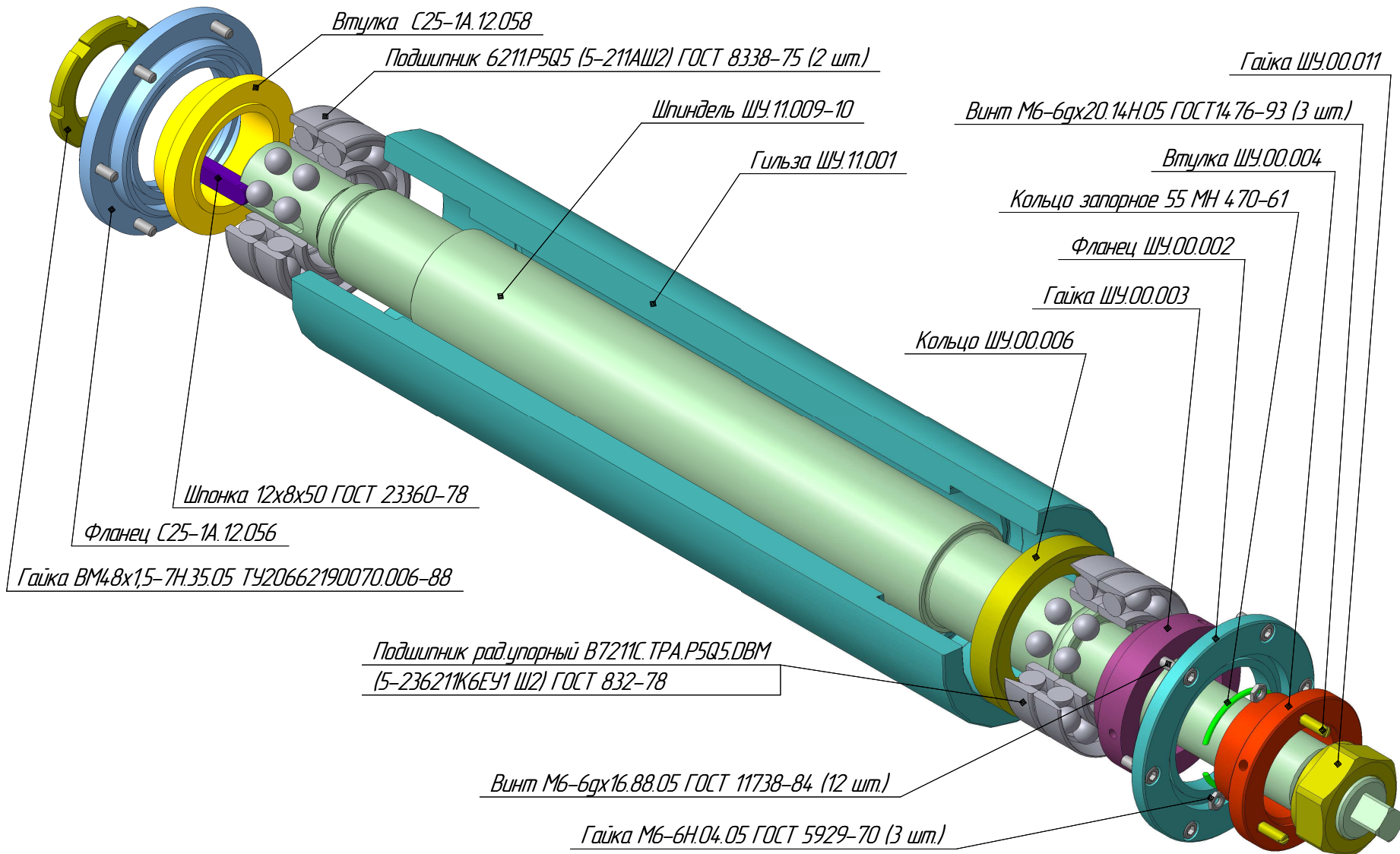
Шпиндель ШУ.11.000-10 СБ (лист 6/6)
