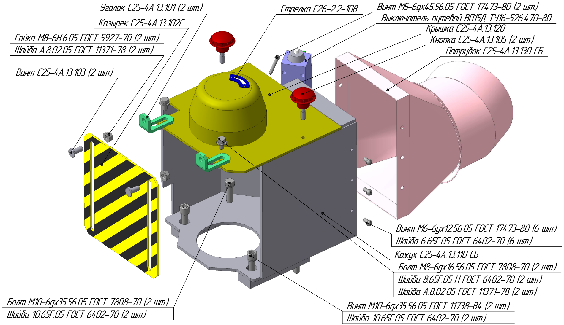
Ограждение С25-4А.13.100 СБ (лист 4/6)
