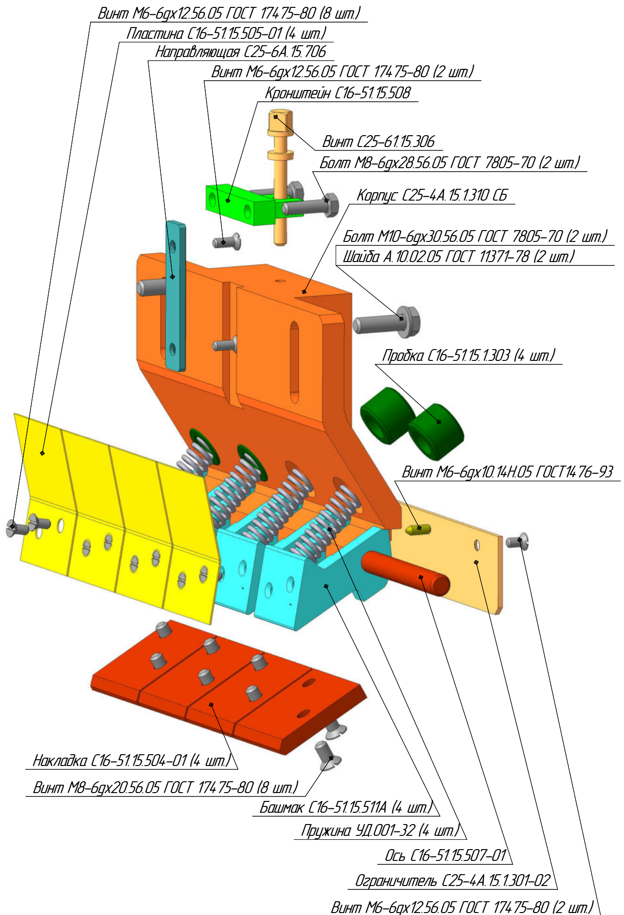
Прижим передний С25-4А.15.1300 СБ (лист 9/13)
